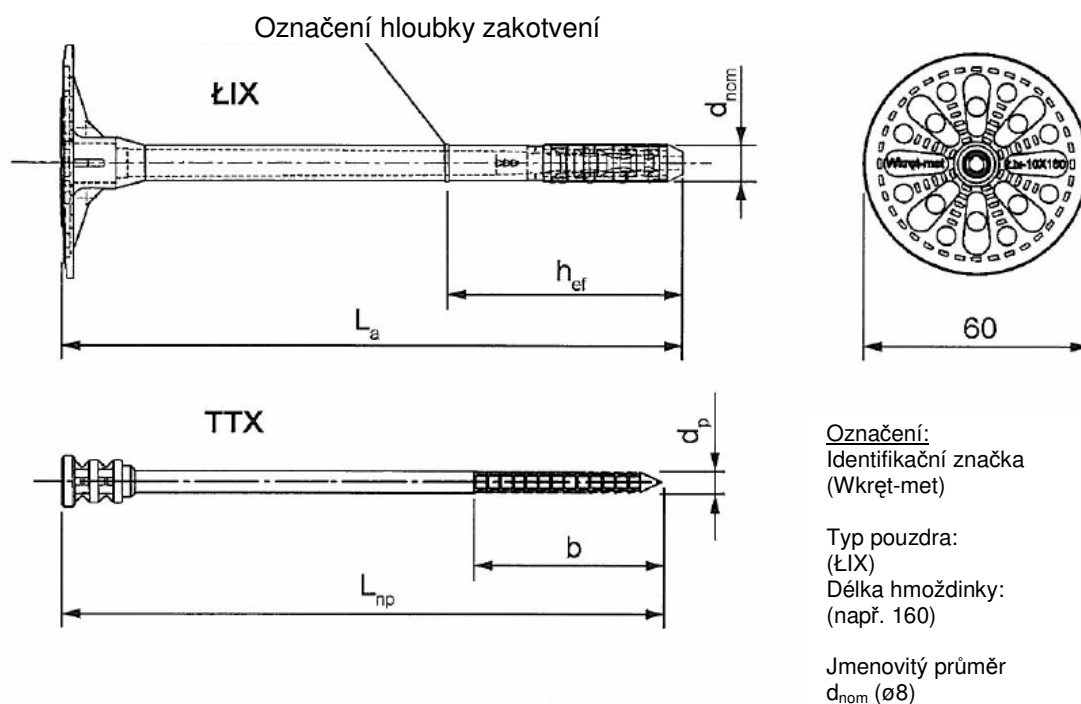
Tabulka 1: Označení a rozměry plastových hmoždinek WKŘET-MET-ŁTXø8 [mm]
