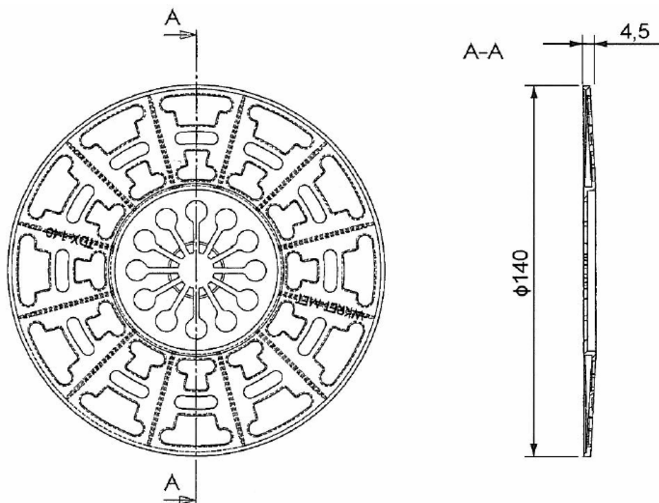
Tabulka 7: Přídavný talířek TDX-140
