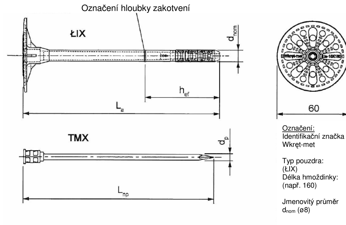
Tabulka 2: Označení a rozměry plastových hmoždinek WKŘEŤ-MET-ŁMXø8 [mm]
